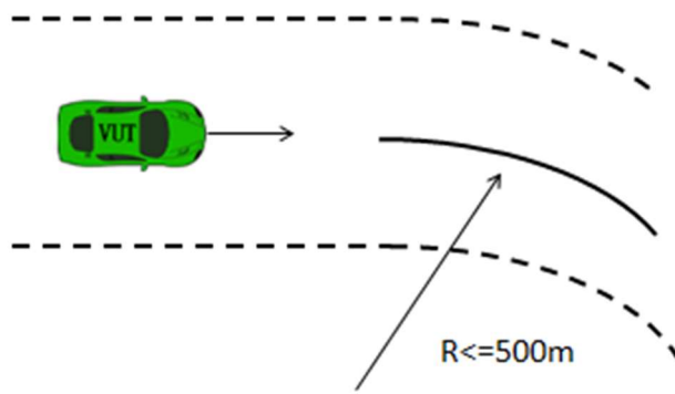
图 6.3 车道线识别及响应测试场景示意图
